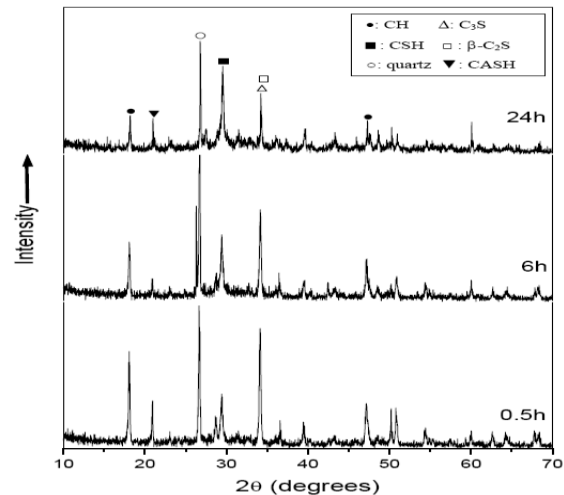
الشكل (3) نتائج تحليل حيود اشعة اكس للعينة الثانية
