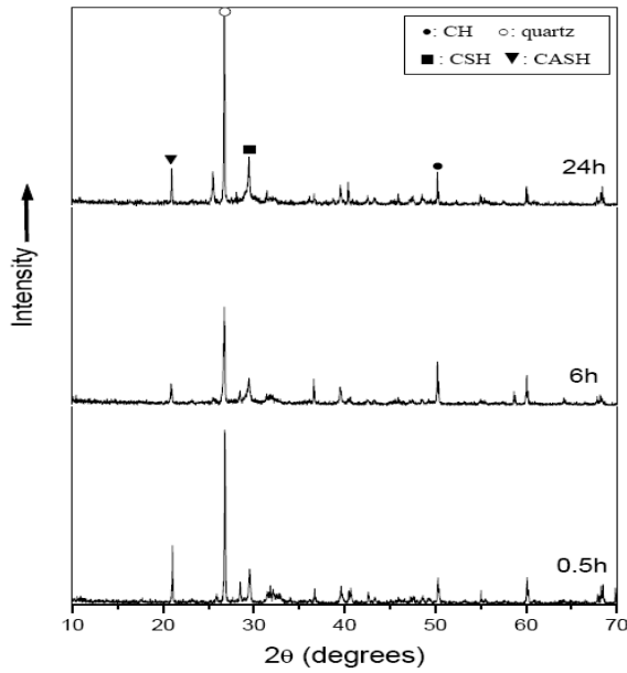
الشكل (2) نتائج تحليل حيود اشعة اكس للعينة الاولى (العينة القياسية)
