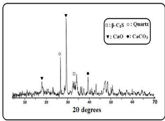
الشكل (1) نتائج تحليل حيود الاشعة السينية للغبار افران الاسمنت .
