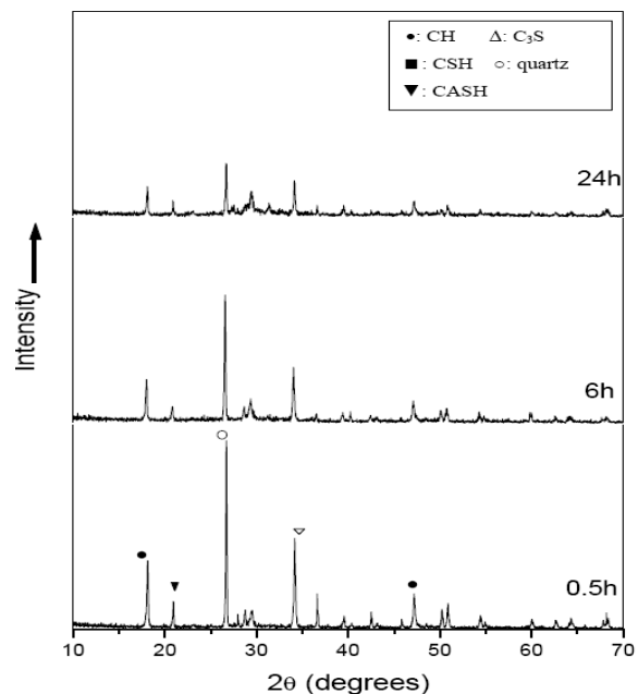
الشكل (4) نتائج تحليل حيود اشعة اكس للعينة الثالثة
