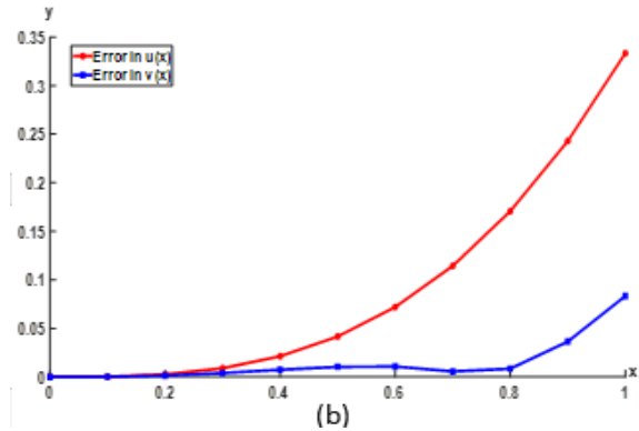
شكل 2 : النتائج العددية للمثال 2: (a) مقارنة بين حلول (VIM) والحلول الفعلية، (b) الخطأ المطلق للمنظومة.
