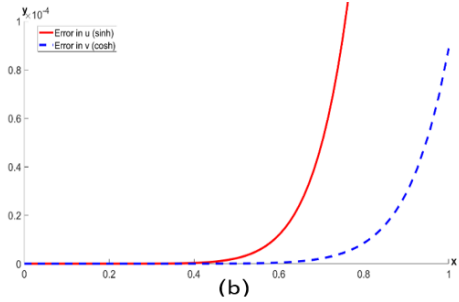
شكل 1 : النتائج العددية للمثال 1: (a) مقارنة بين حلول (VIM) والحلول الفعلية، (b) الخطأ المطلق للمنظومة.
