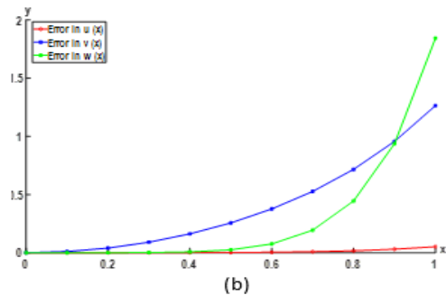
شكل 4 : النتائج العددية للمثال 4: (a) مقارنة بين حلول (VIM) والحلول الفعلية، (b) الخطأ المطلق للمنظومة.
