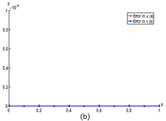
شكل 3 : النتائج العددية للمثال 3: (a) مقارنة بين حلول (VIM) والحلول الفعلية، (b) الخطأ المطلق للمنظومة.
